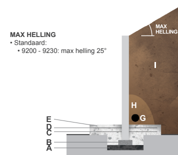
Belastingsschema klasse B
