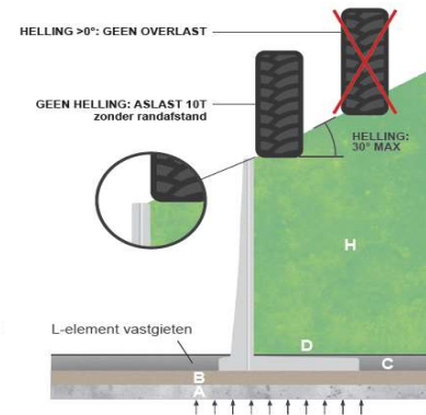
Belastingsschema Klasse C Silo 1
