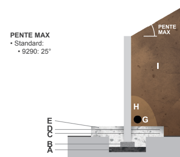
Classe de charge B
